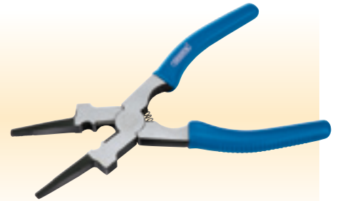
5 WP1 210mm MIG 'Helper' Pliers
